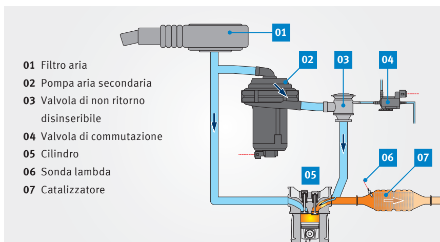
Principio dell'iniezione aria secondaria (ad azionamento pneumatico)
