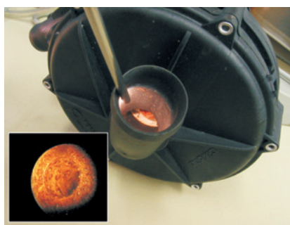
Sguardo nel bocchettone corrosivo di una pompa aria secondaria
